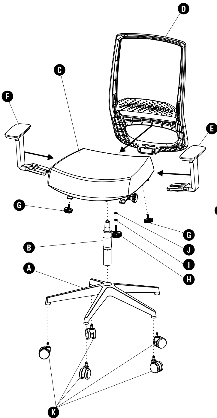
Deluxe Mechanism Shown Mécanisme de luxe illustré Mecanismo de lujo mostrado
